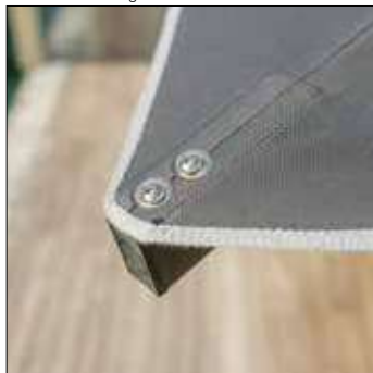
canvas fixing system fixation de la couverture du parasol sistema de fijación de la lona
